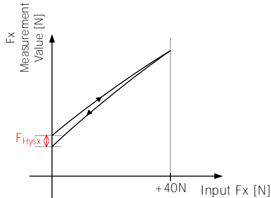
Fig. 6 Hysteresis (e.g.: Fx)
