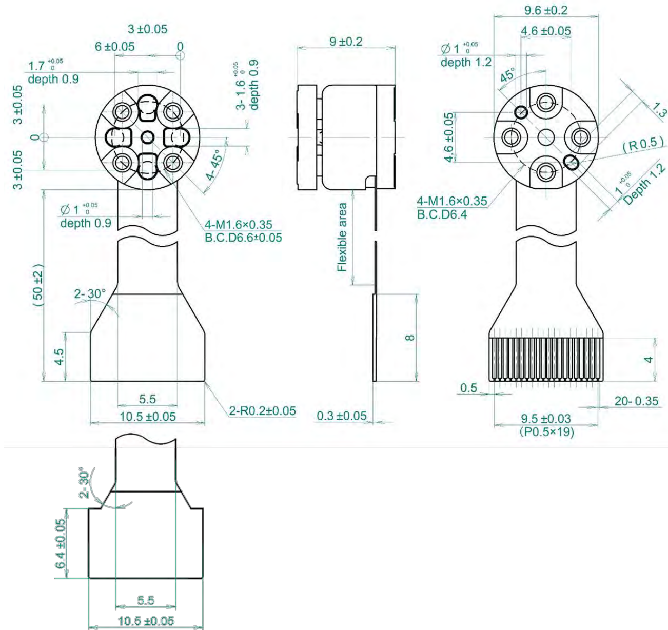
Fig. 26 Dimensions
